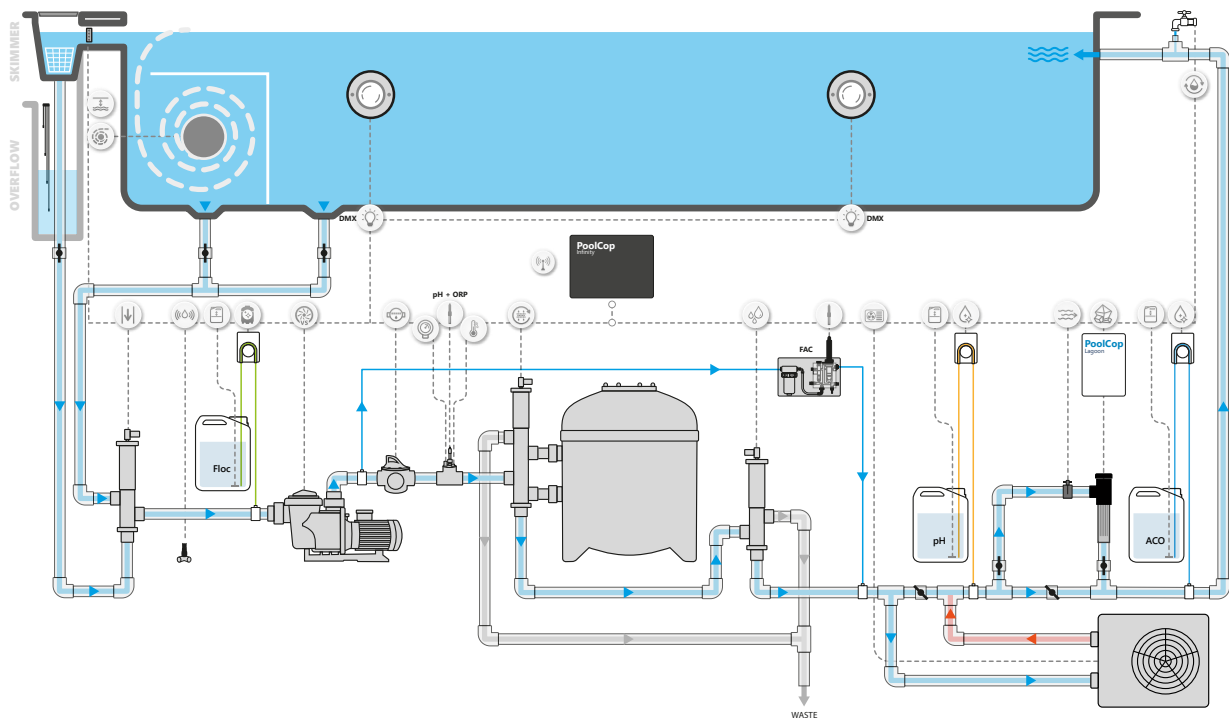
POOLCOP INFINITY - POMPE UNIQUE AVEC ACQUISITION DE DONNÉES, AUTOMATISATION & DÉSINFECTION AU SEL
