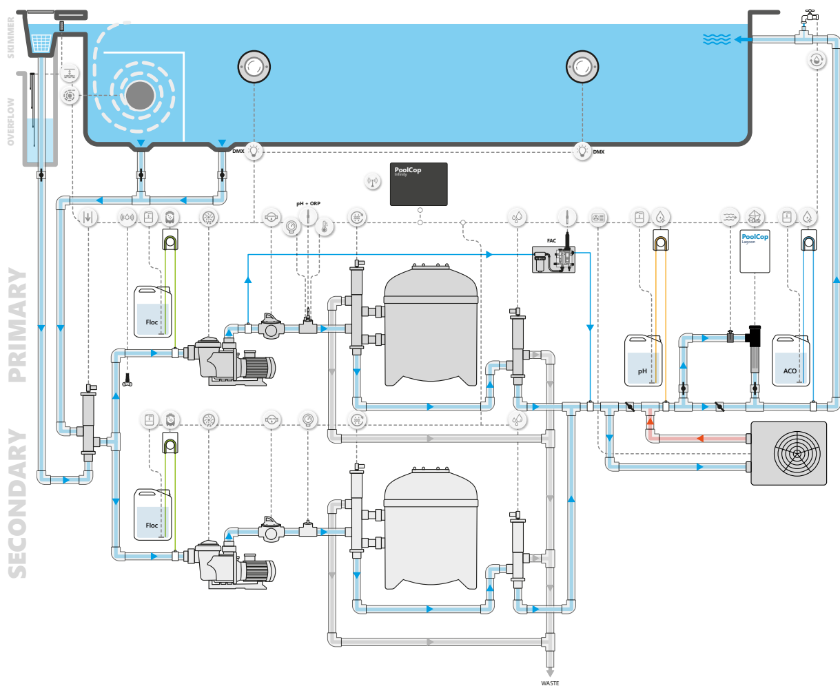
POOLCOP INFINITY - DEUX POMPES AVEC ACQUISITION DE DONNÉES, AUTOMATISATION & DÉSINFECTION AU SEL
