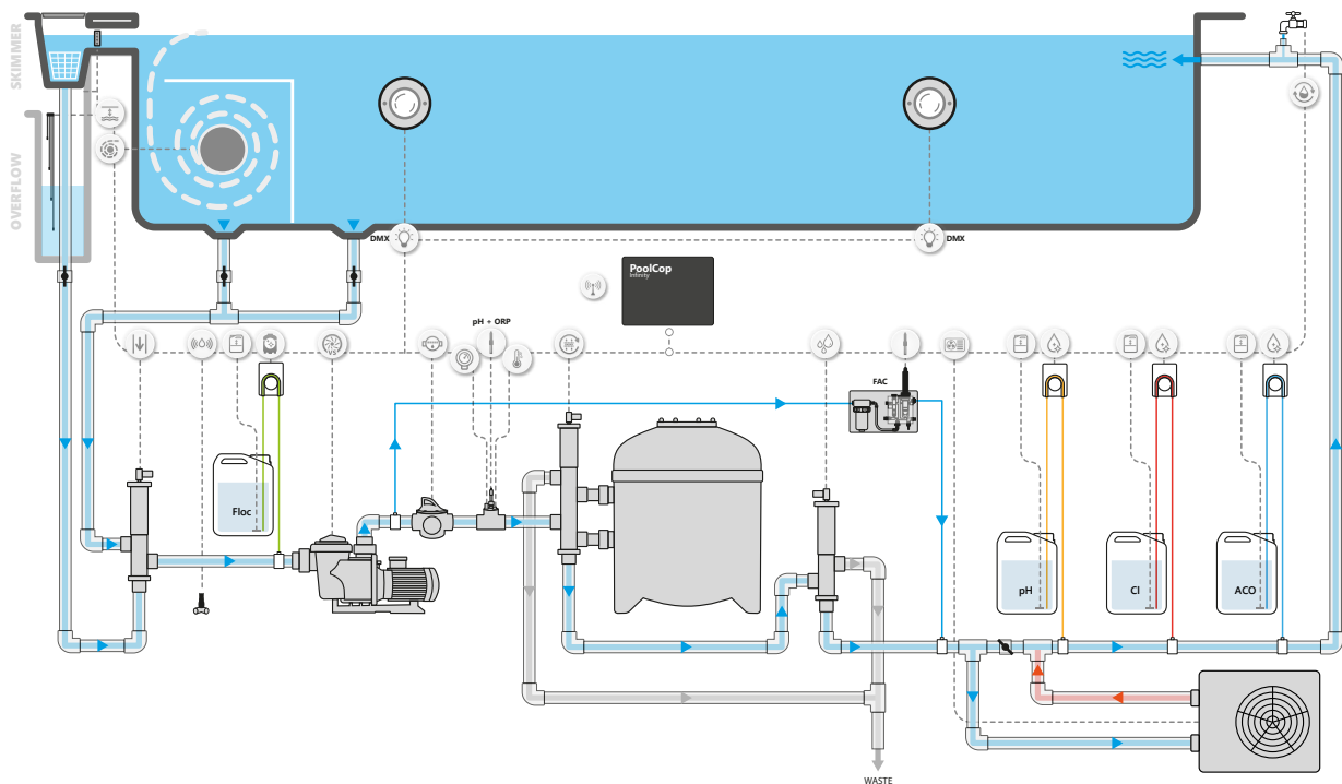
POOLCOP INFINITY - POMPE UNIQUE AVEC ACQUISITION DE DONNÉES, AUTOMATISATION & DÉSINFECTION AU CHLORE
