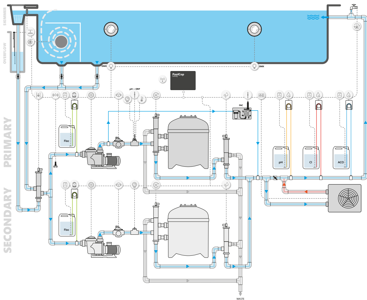
POOLCOP INFINITY - DEUX POMPES AVEC ACQUISITION DE DONNÉES, AUTOMATISATION & DÉSINFECTION AU CHLORE
